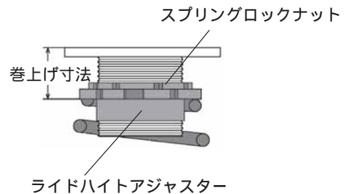
【ライドハイトアジャスターASSY】
